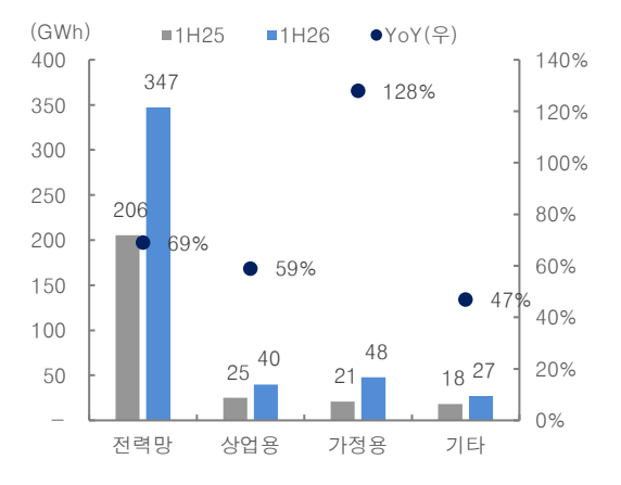
그림 119. 용도별 ESS 배터리 출하
