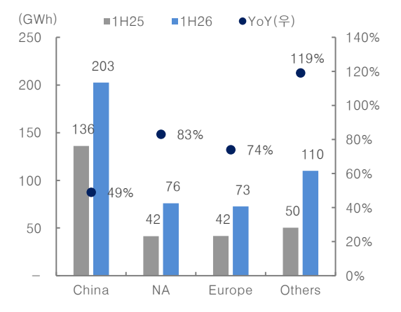
그림 117. 지역별 ESS 배터리 출하
